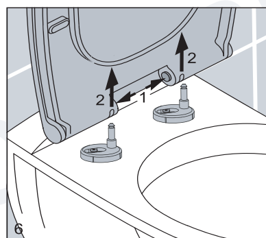
6 Retirer le siège et le couvercle des toilettes en appuyant sur les deux boutons-poussoirs
