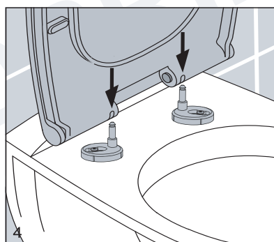
4 Clip sur le siège et le couvercle des toilettes
