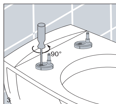
3 Desserrer légèrement les vis en les tournant à 90° vers la droite
