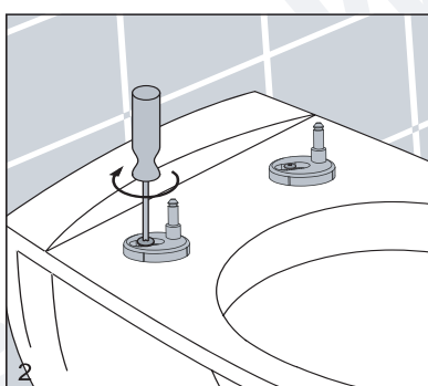
2 Serrer les vis des charnières
