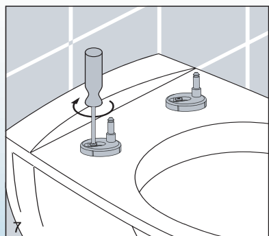
7 Serrer les vis
